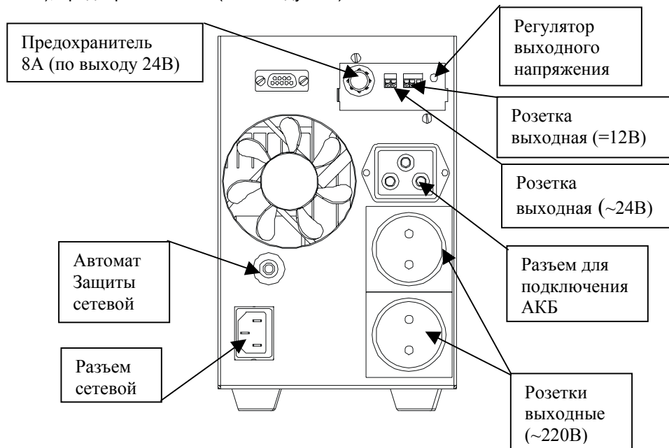
Рис. 2 Задняя панель блока
