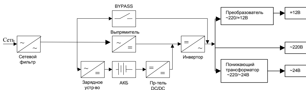
Рис. 3 Структурная схема ИБП
