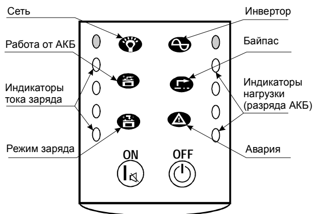
Рис. 1 Передняя панель блока ИБП
