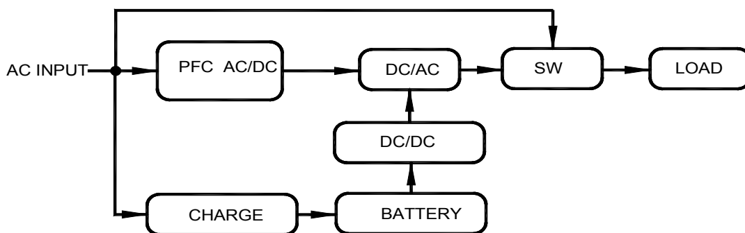
Рис.3.1-1 Блок-схема ИБП Monolith K 6000LT
