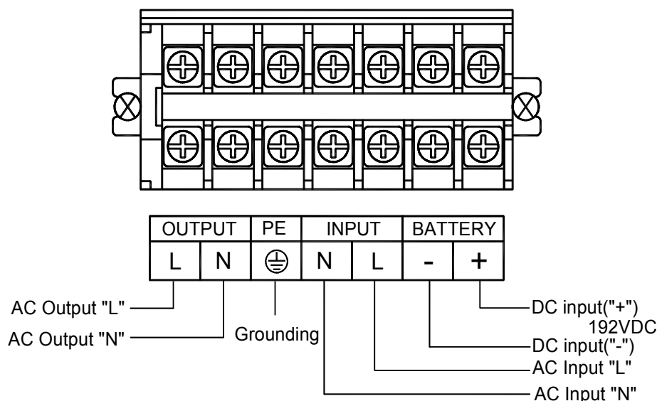
Рис. 4.8-1 Клеммная колодка ИБП Monolith K 6000LT
