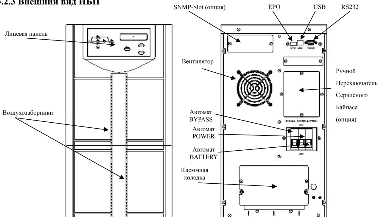
Рис.3.3-3 Внешний вид ИБП Monolith K 6000LT
